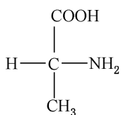
D-丙氨酸
