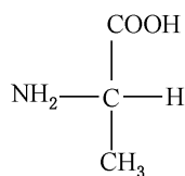
L-丙氨酸
